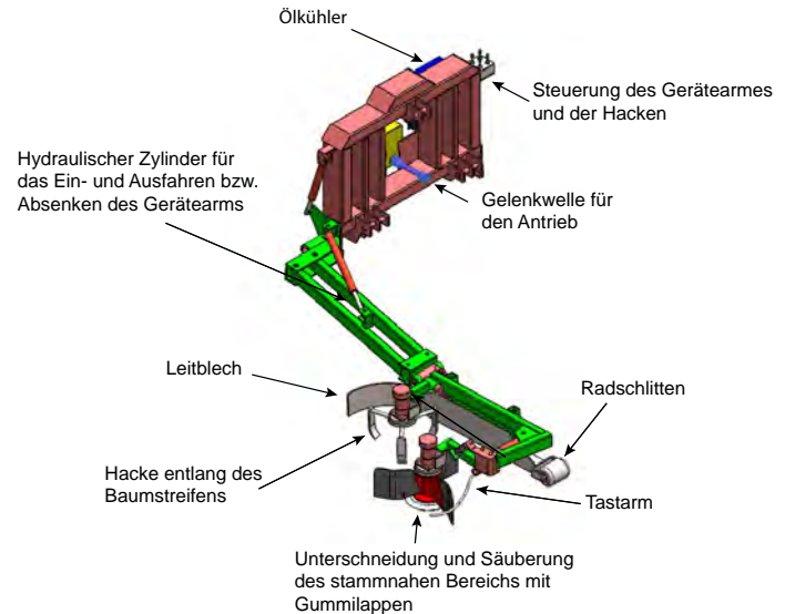
Abb. 16: Krümler/Unterstockbearbeitungsgerät
