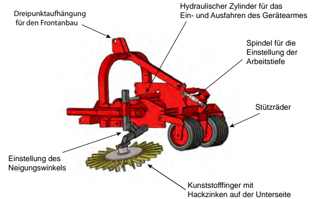
Abb. 14: Fingerhacke an Mehrgerätenbauahmen
