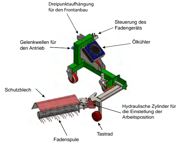
Abb. 20: Fadengerät
