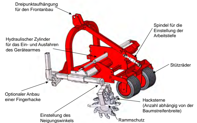
Abb. 12: Rollhacke an Mehrgerätenaurahmen
