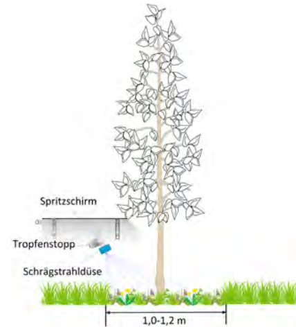
Abb. 4: Schematische Darstellung zur Applikation von Herbiziden
