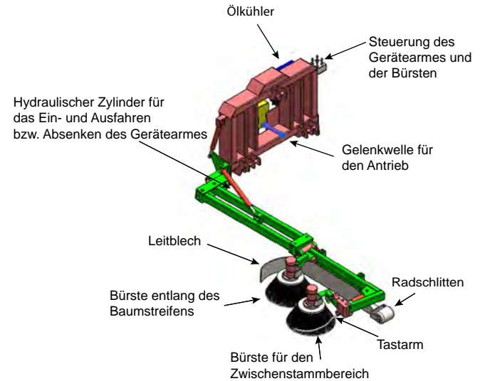
Abb. 22: Vertikales Bürstengerät
