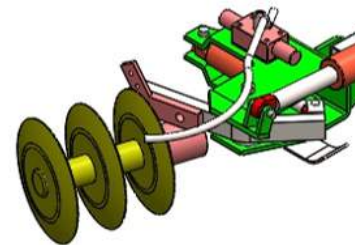
Abb. 19: Scheibenkopf zum Abhäufeln
