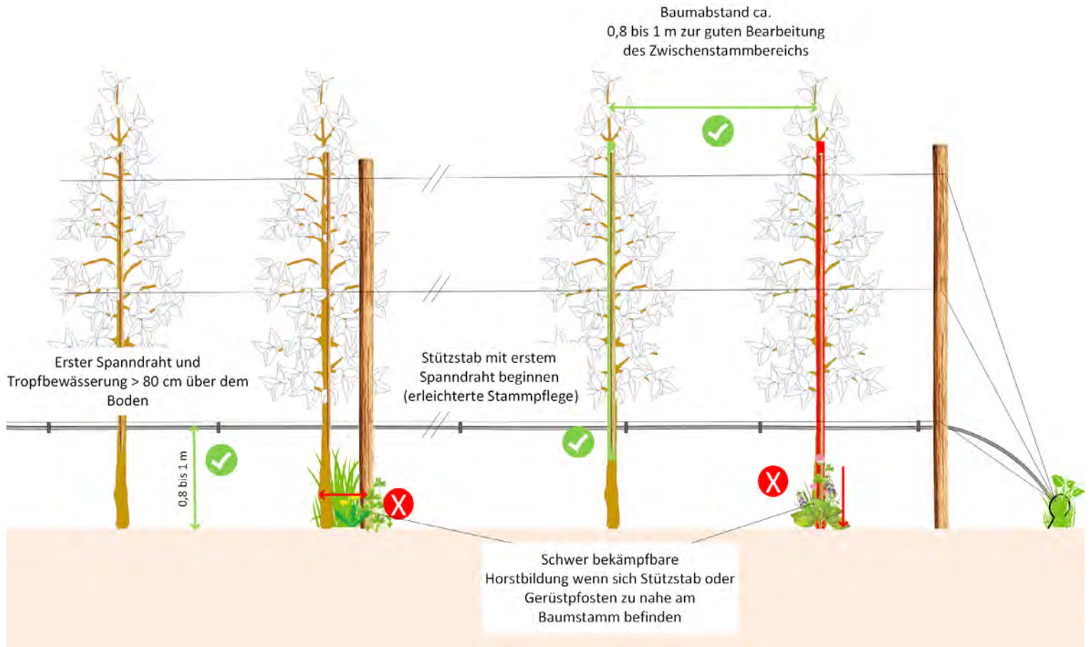
Abb. 10: Gerüstaufbau für die mechanische Beikrautregulierung
