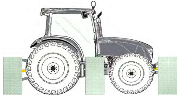
Abb. 6: Anbauräume für mechanische Systeme zur Beikrautregulierung
