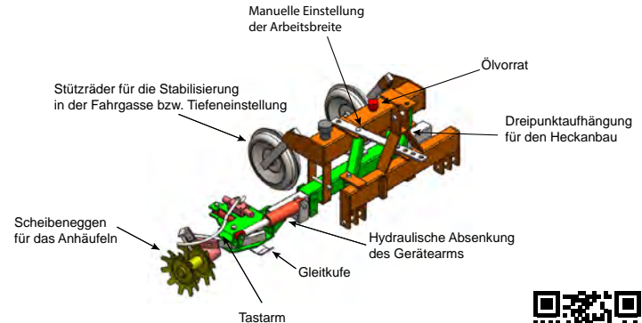
Abb. 18: Scheibenegge zum Anhäufeln
